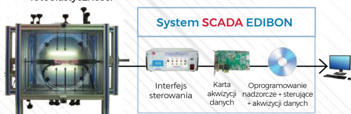
EFOC. Sterowana komputerowo jednostka fotoelastyczności
