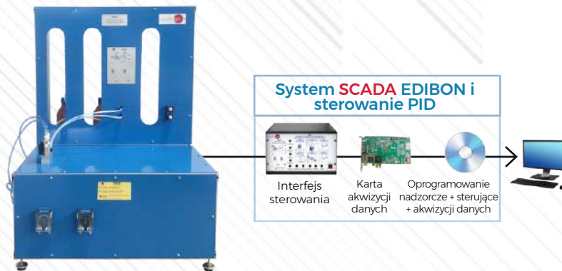
QUSC. Jednostka serwisowa dla QRC
