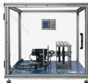
MESE. Jednostka napędowa z przekładnią zębatą
